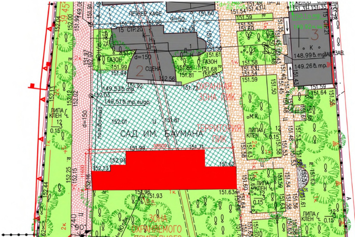
Месторазмещение НТО №1 на генеральном плане участка
